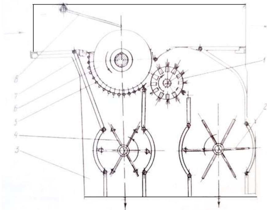
2-rasm. Jinlangan paxta chigitini linterlash jarayonida olinadigan momiqni mayda va yirik iflosliklardan tozalash uchun tavsiya etilayotgan aeromexanik momiq tozalagichini konstruktiv sxemasi
